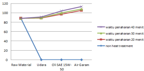
Gambar 5. Grafik Hasil Pengujian Kekerasan (HRB)
