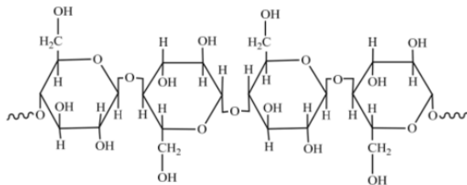
Gambar 3. 1 Struktur Selulosa
