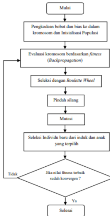
Gambar 2 Diagram Alir Optimasi Bobot Backpropagation dengan GA (BPNGN)
