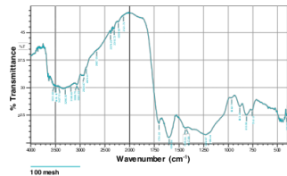
Gambar 2. Grafik uji FTIR sampel ukuran 100\text{ mesh}
