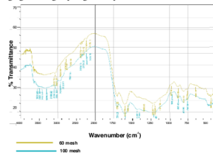
Gambar 3. Grafik uji FTIR sampel ukuran 60\text{ mesh} dan 100\text{ mesh}
