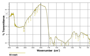
Gambar 1. Grafik uji FTIR sampel ukuran 60 mesh
