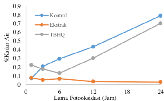
Gambar 6. Grafik Hasil Pengukuran Kadar Air
