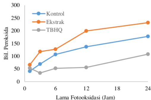
Gambar 5. Grafik Hasil Penetapan Bilangan Peroksida
