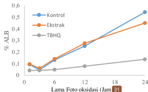
Gambar 4. Grafik Hasil Pengukuran Kadar Asam Lemak Bebas
