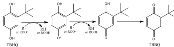
Gambar 4. Reaksi Oksidasi TBHQ Membentuk TBBQ.
