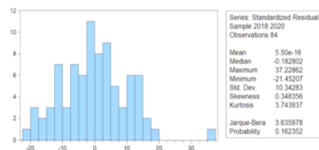
GAMBAR 2. Hasil Uji Normalitas
